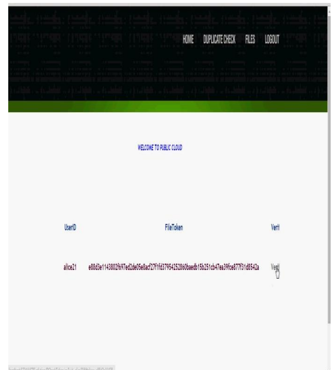
Fig: 5 Data
