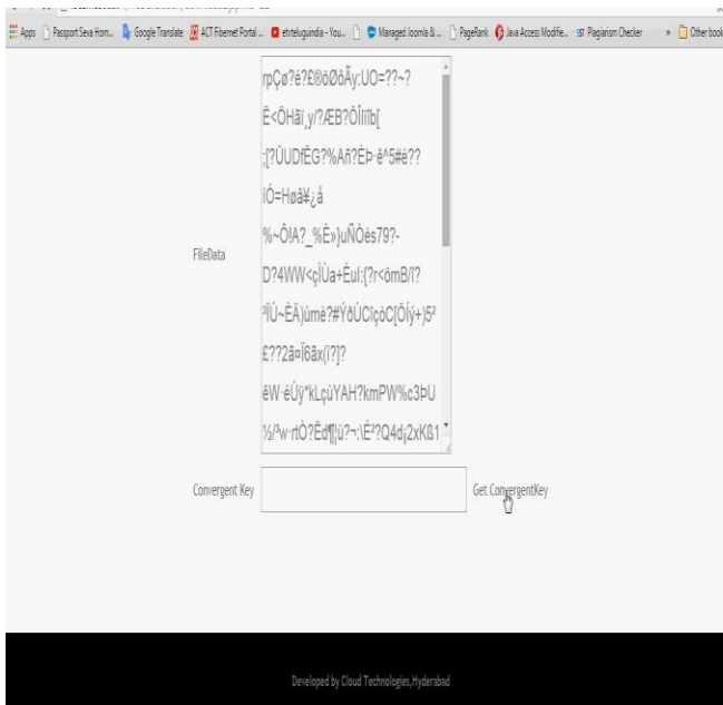
Fig: 6 Encryption
