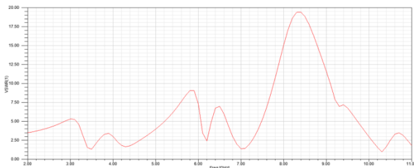
Fig. 7 VSWR
